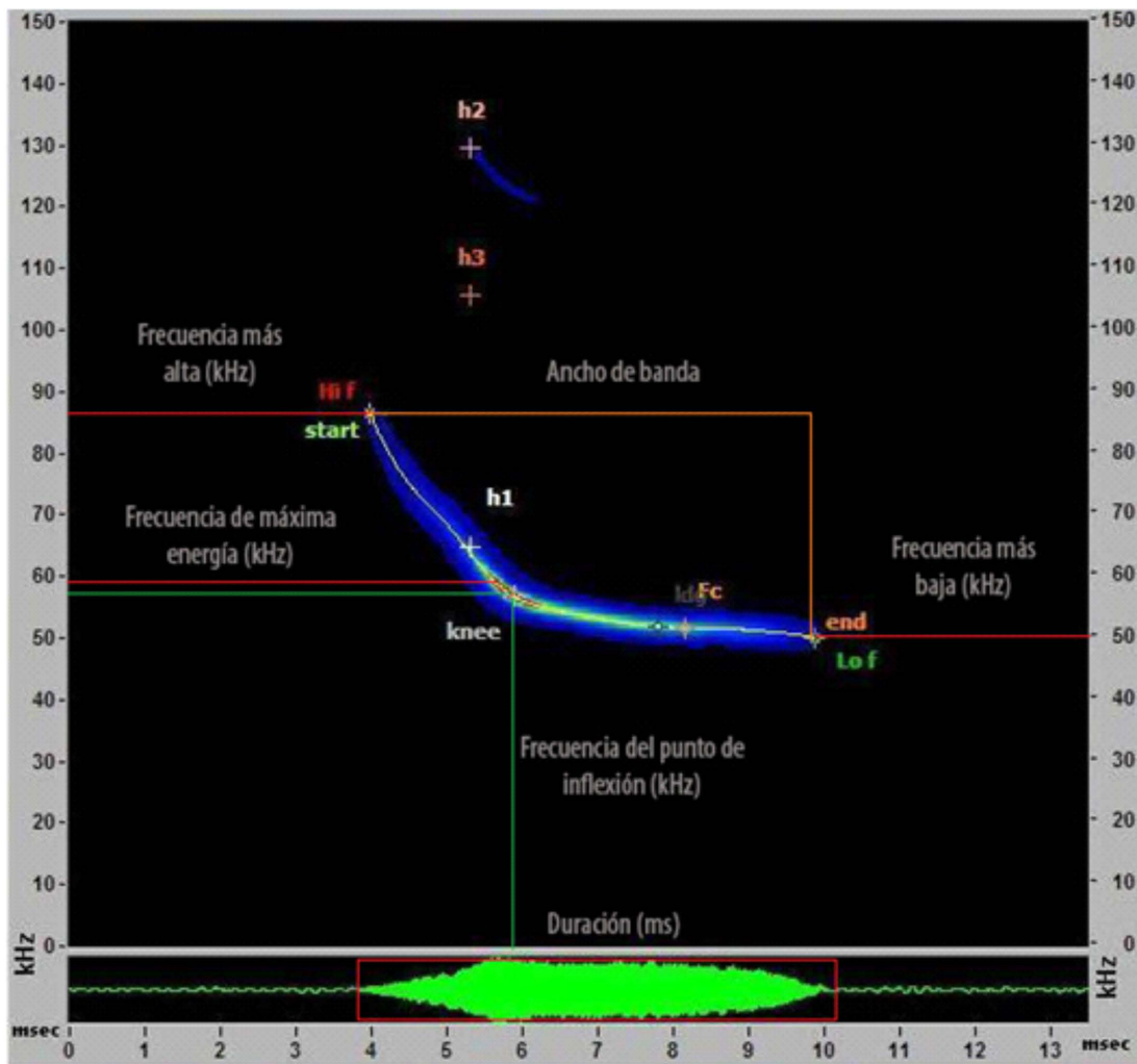
Figura 2. Parámetros medidos de las diferentes llamadas, frecuencia más alta ( Hif ), frecuencia más baja ( Lof ), frecuencia inicial ( start ), frecuencia final ( end ), frecuencia del punto de inflexión ( knee ), número de armónico ( h1 ), frecuencia característica ( Fc ), parte de la llamada con la mayor intensidad ( kd ), duración y ancho de banda.
